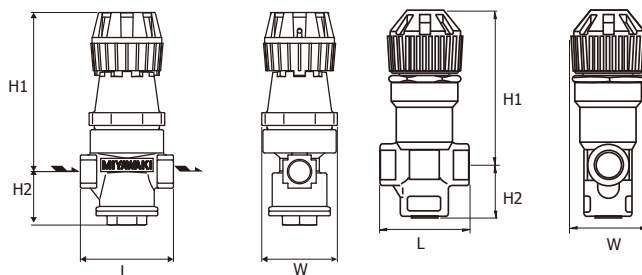
Dimensions RE1
