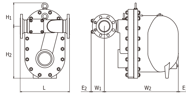
Dimensions GH70
