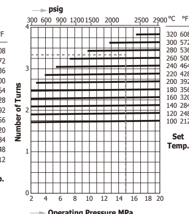
TBH82 - 200
