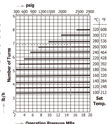
TBH81 - 200
