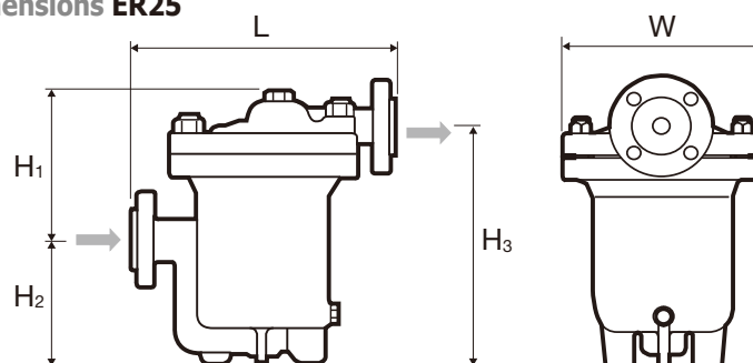
Dimensions ER25
