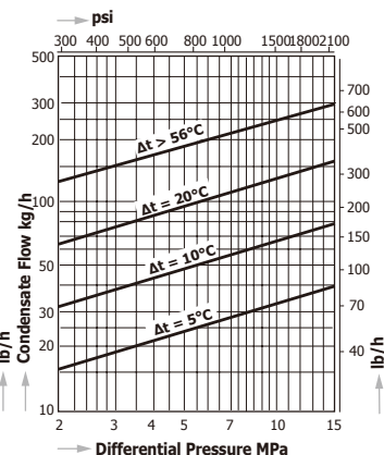
TBH82 - 200
