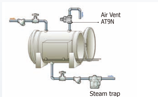
Autoclave
