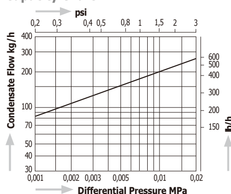
Capacity Chart F1
