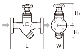
SV - 4NF, 6NF, 8NF
