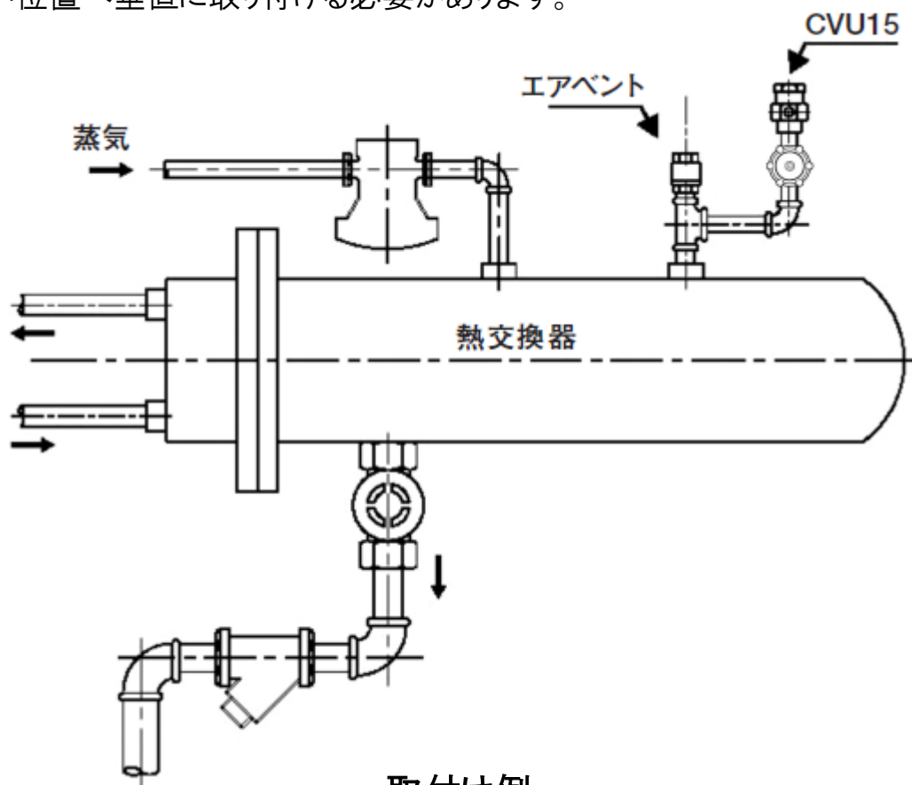
取付け例
