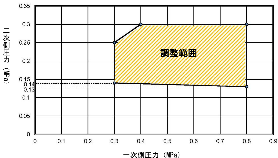
RE1LM型 調整圧力範囲
